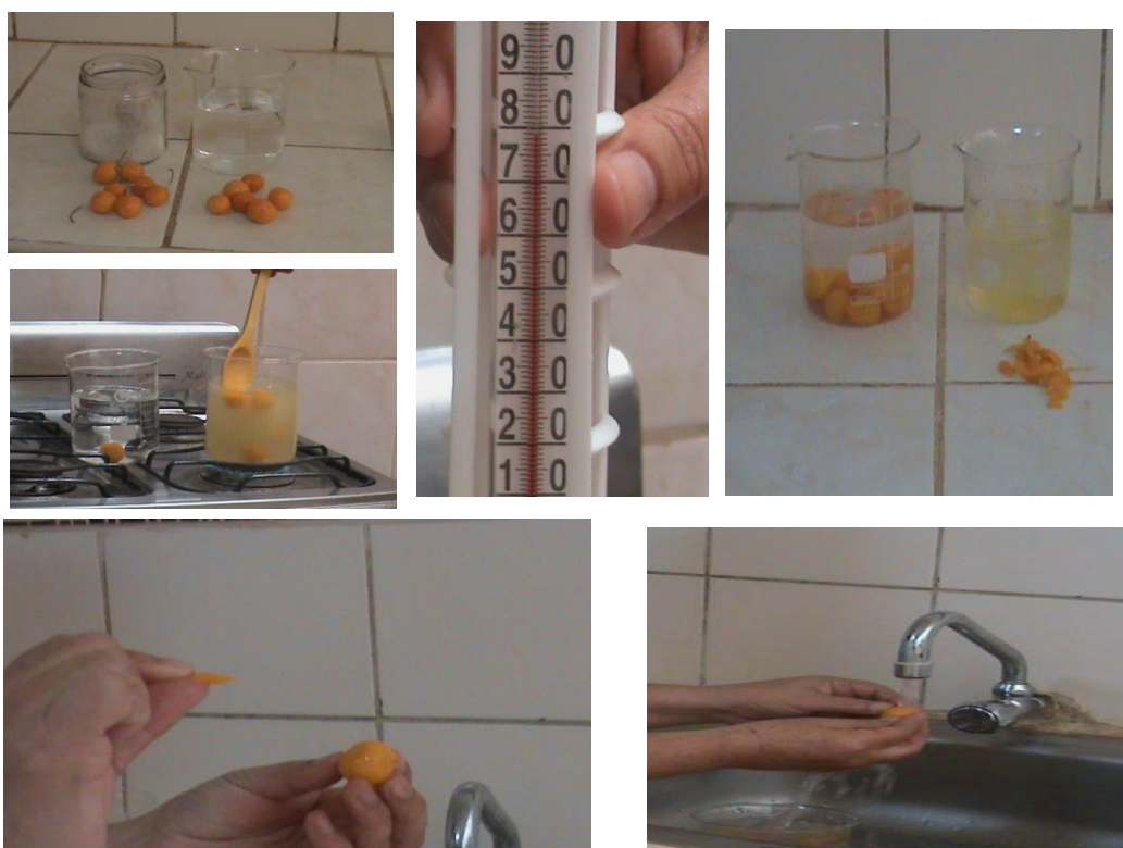
Figura 5: Pelado químico del Aguaymanto
